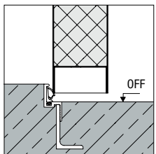
Anschlagschiene mit Dichtung
