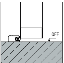
Aufgesetzte Anschlag-schiene mit Dichtung
