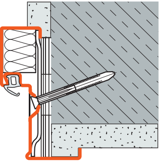
Diagonalbefestigung (Mauerwerk)
