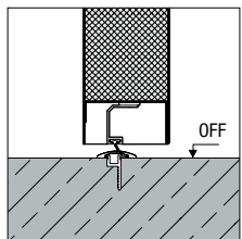
Aluminium-Abschluss-profil mit Dichtung
