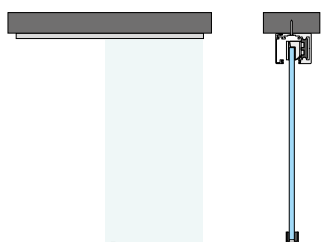
Deckenmontage
