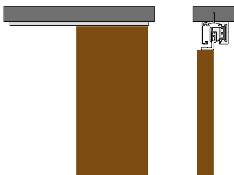
Deckenmontage
