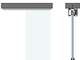
Deckenmontage
