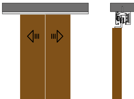
Deckenmontage
