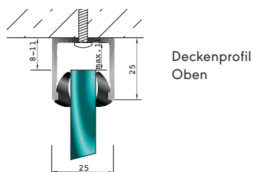
U-Profil mit Clip Profil (Gummi Transparent)
