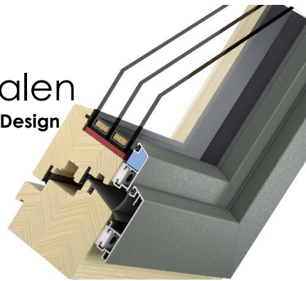
SOLID(Flächenversetzt)
