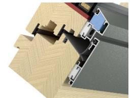
FLAT (Flächenbündig)
